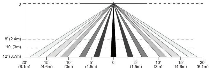
Lente de alta densidad o de alcance reducido CI-24-1 Vista lateral
